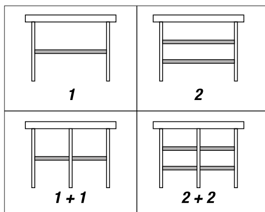
Variety příčných vzpěr
