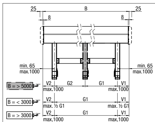
B = celková šířka (bez bočních krytů PS619/.)
