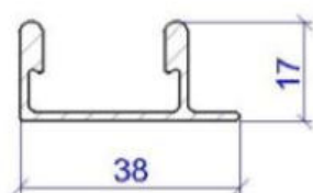
NÁKRES INTERIEROVÉ KOLEJNÍČKY
